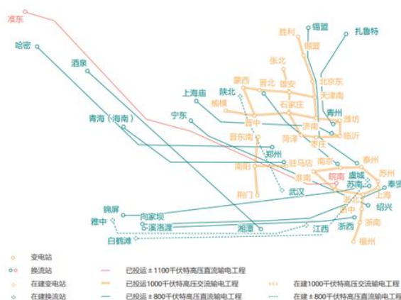
图36: 建成及在建特高压线路图
